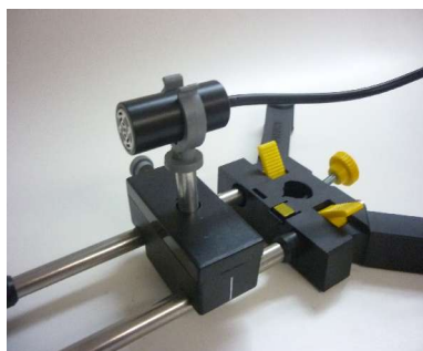
Montage guide pour les Ultras Sons
